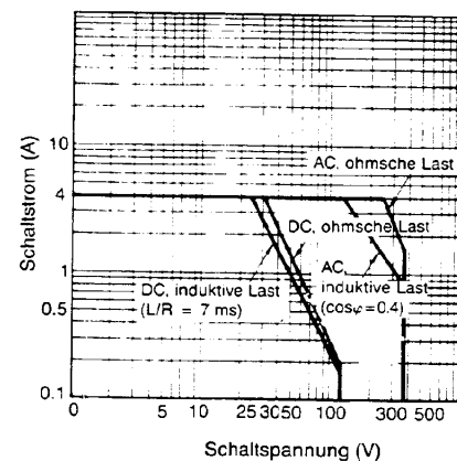
zweipoliger, waschdichter Typ G2R-2(A)4
