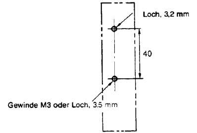
Anordnung der Anschlüsse (Ansicht von oben)
