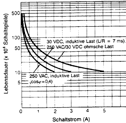
einpoliger Hochleistungstyp G2R-1(A)-E
