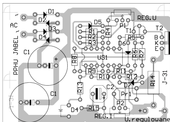
Obrázek plošného spoje
